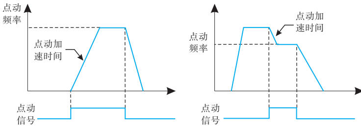
图6-05 点动运行
