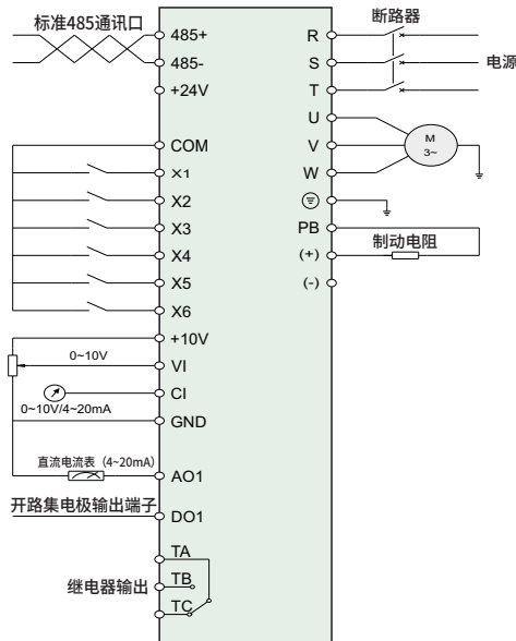
图3-4 基本配线图
