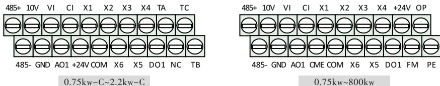
图3-8 控制板端子排列顺序图
