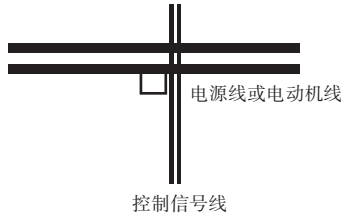
图3-17 系统配线要求
