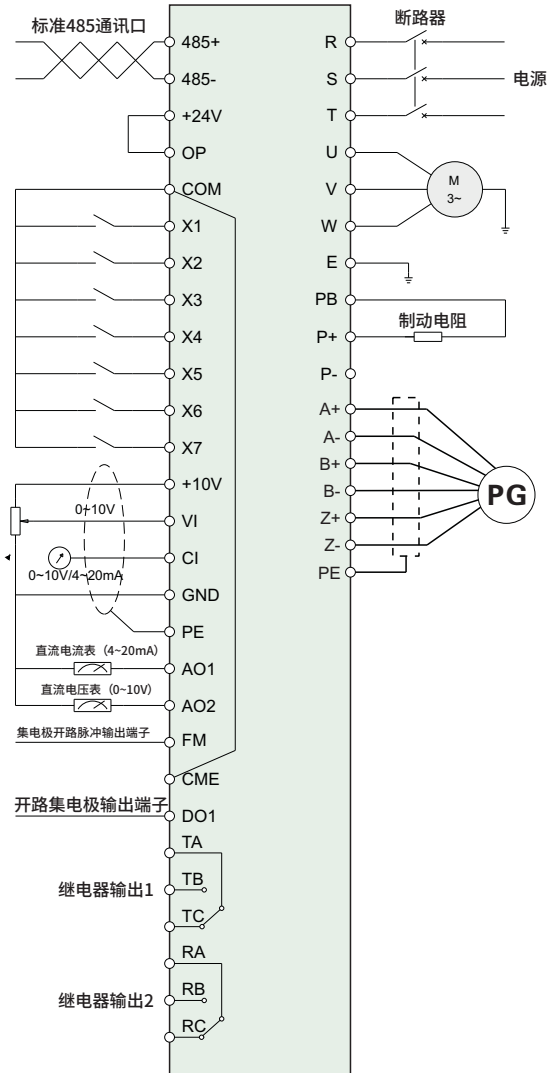
图3-6 基本配线图 (WD990-4T0300G, WD990-4T0370G)
