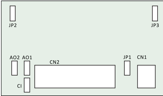
图3-7 控制板端子跳线位置示意图
